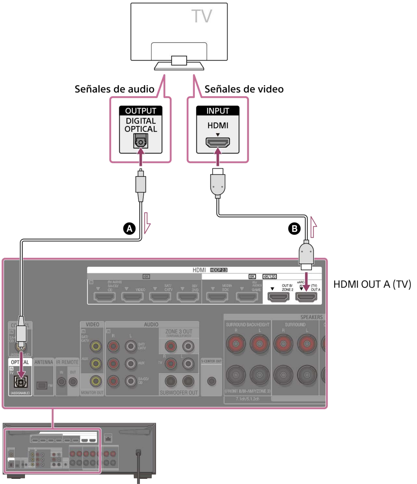
Conexión con un cable HDMI y un cable de audio
