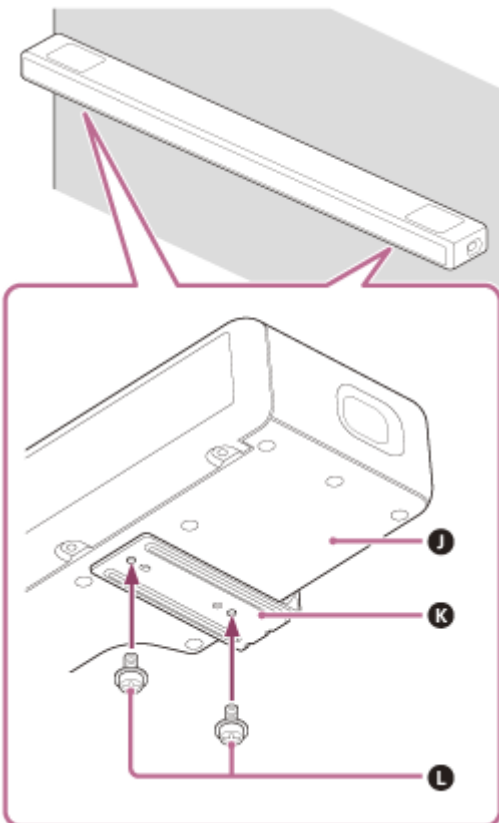
J Нижняя часть звуковой панели
