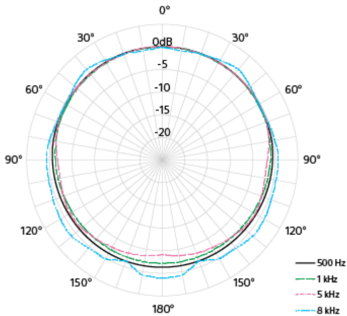
Частотна характеристика в неспрямованому режимі
